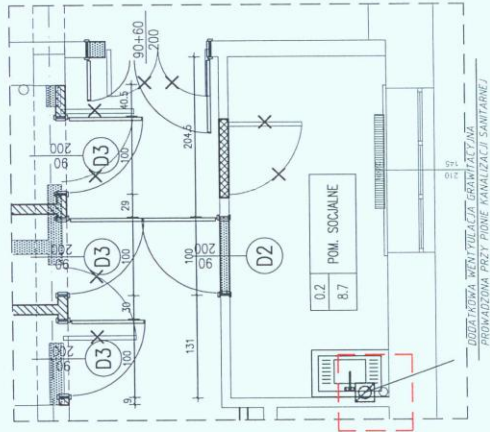
FRAGMENT PARTERU SKALA 1:50
